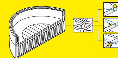
Beispielhafte Illustration eines HEPA-14-Filter
